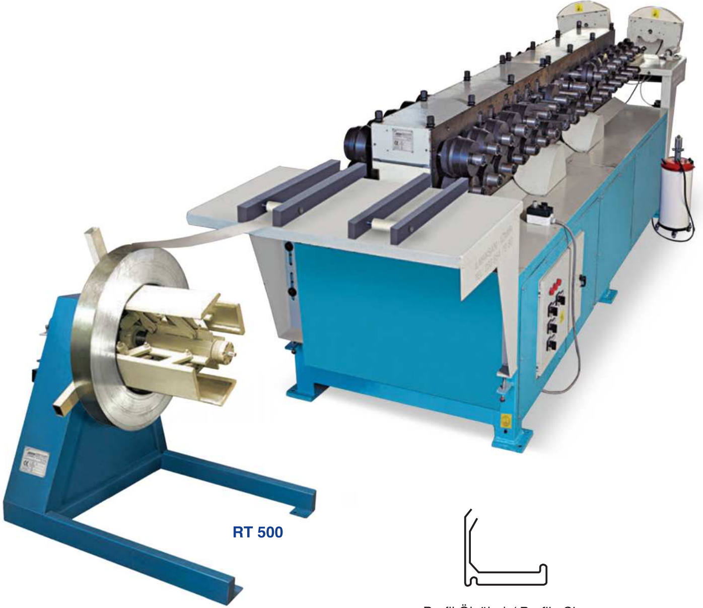
Profil Ölçüleri / Profile Size 20 - 25 - 30 - 35
